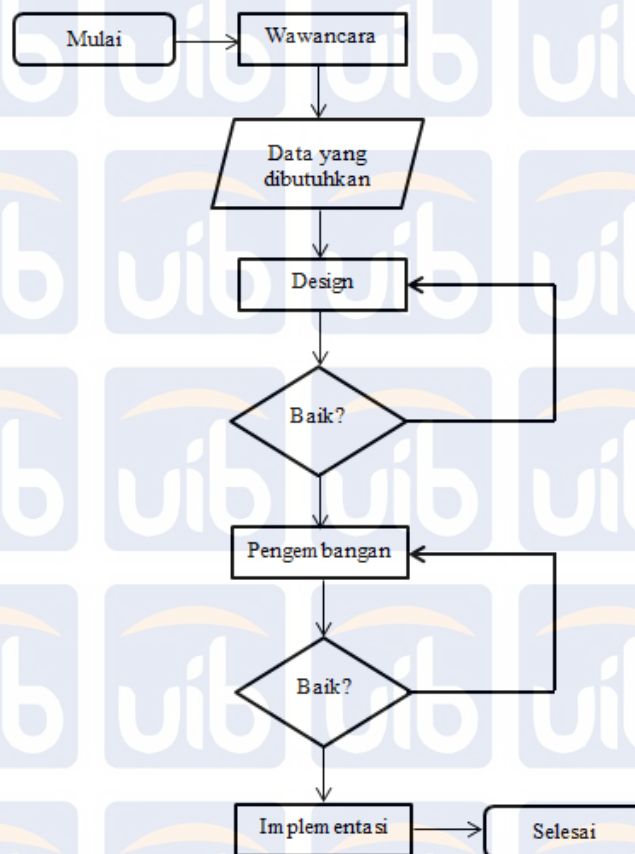
Gambar 1 Proses Perancangan
