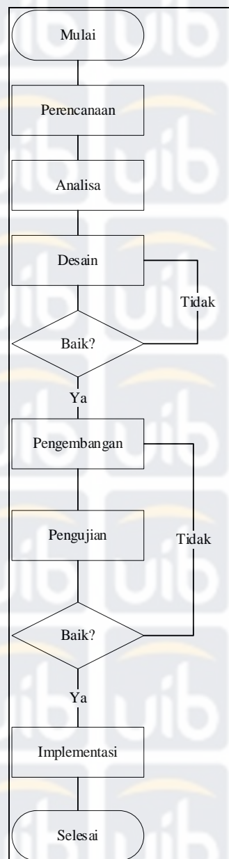
Gambar 2 Flowchart proses perancangan sistem
